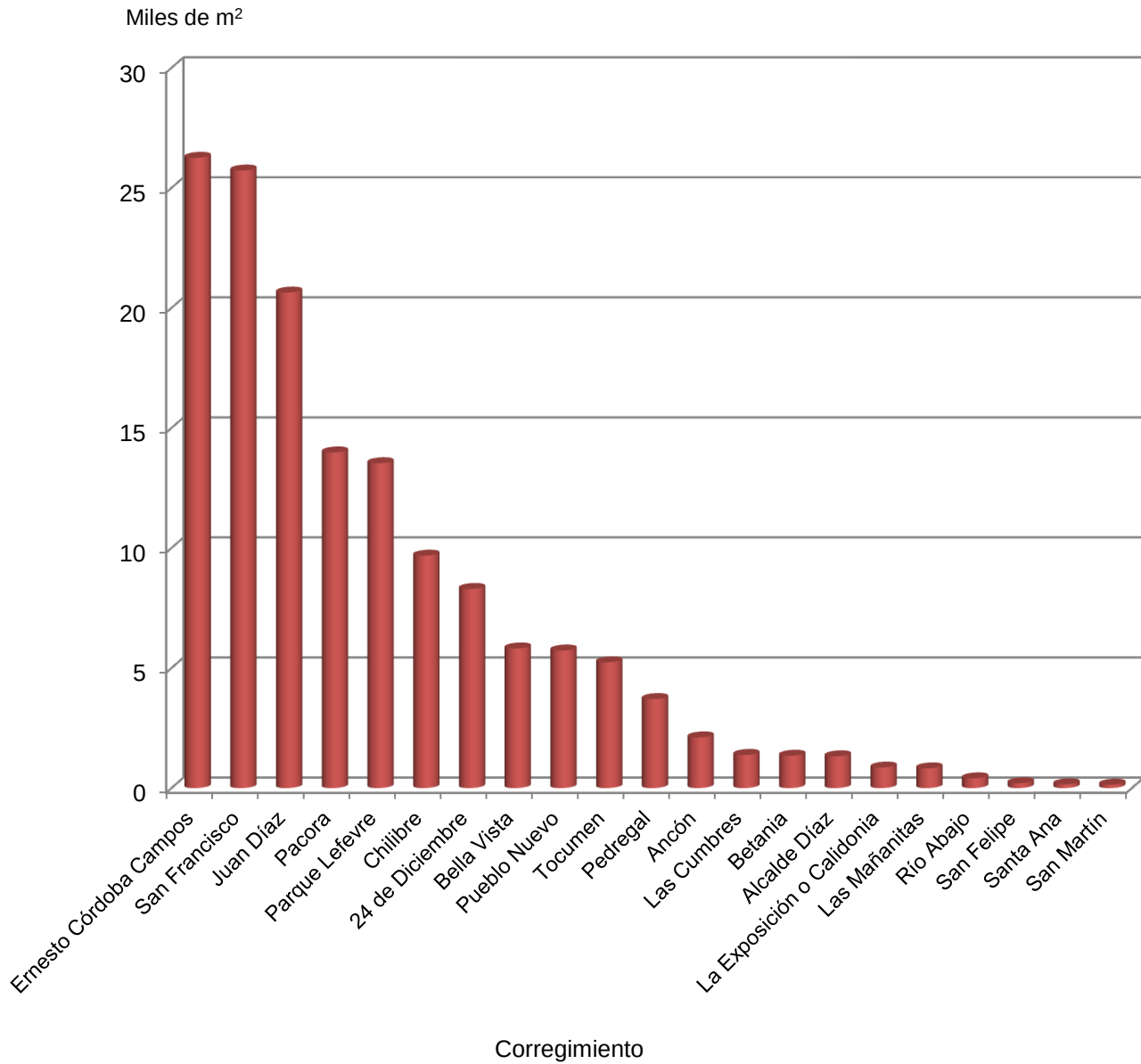
Gráfica 3. CONSTRUCCIONES EN PROCESO EN EL DISTRITO DE PANAMÁ, POR ÁREA CONSTRUIDA, SEGÚN CORREGIMIENTO: PRIMER TRIMESTRE DE 2016 (P)
